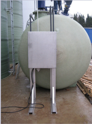
Liuosaseman sähkökeskus
