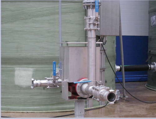
Varastosäiliön pumppausputkisto
